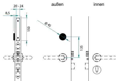
Abmessungen Leser und Elektronik
